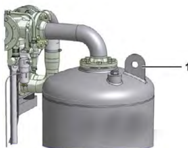
Zdvíhacie oká a upevňovacie oká na nádržiach
