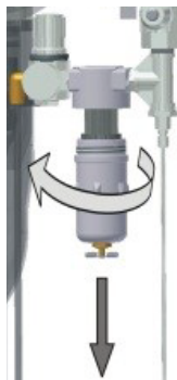
Otvorenie filtra riadiaceho vzduchu
