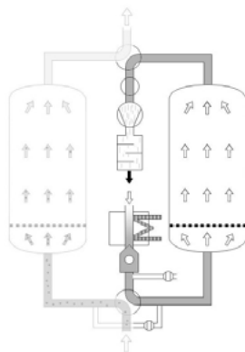
Fáza vykurovania
