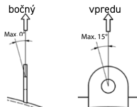
Preprava žeriavom
