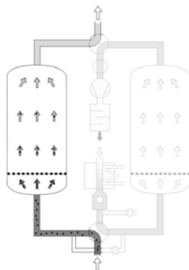
Adsorpcia, tu zobrazená v ľavej nádrži
