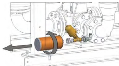
Uvoľnenie tlmiča hluku
